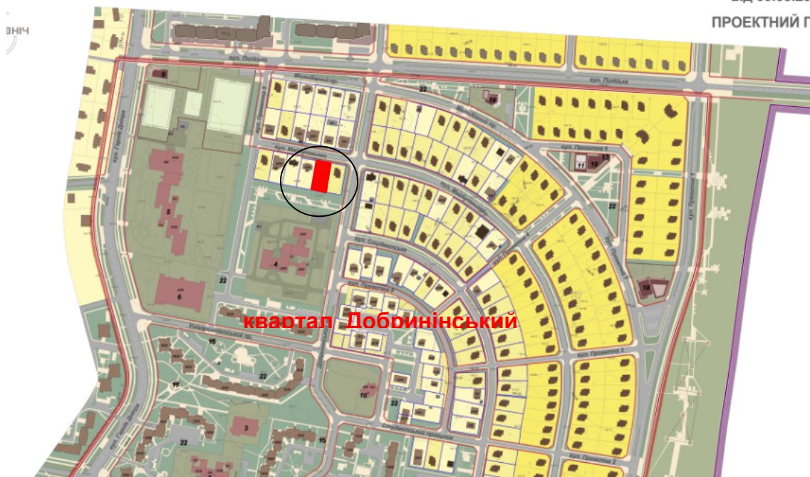
Викопіювання з детального плану кварталу Добринінський м. Славутича
